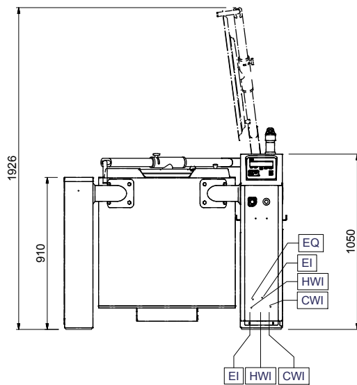
Zij aanzicht
